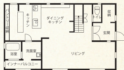
1階
